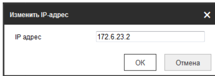
Рисунок 6-18 Изменение IP-адреса
