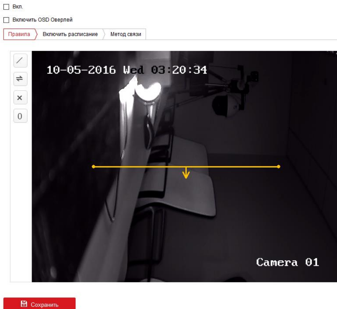
Рисунок 10-34 Настройка подсчета
