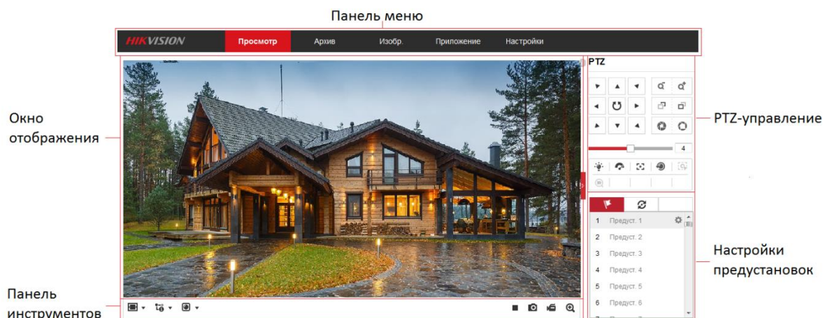
Рисунок 5-1 Интерфейс отображения
