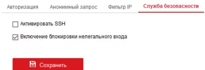
Рисунок 6-19 Служба безопасности
