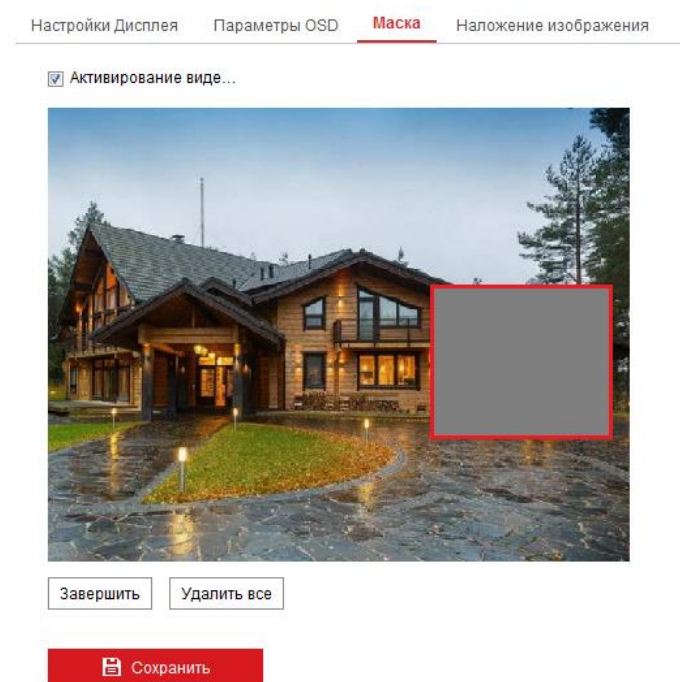
Рисунок 9-7 Настройки маски
