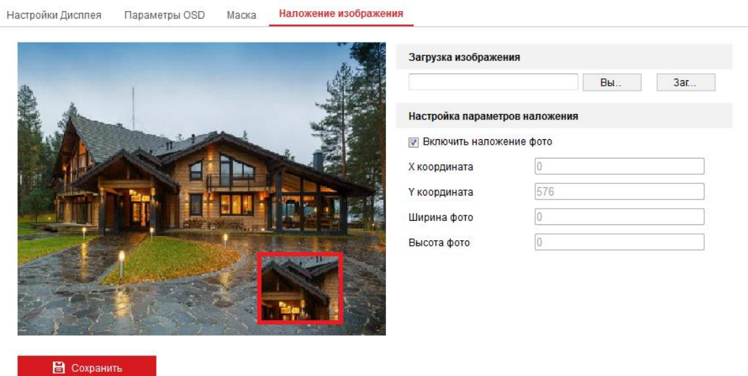
Рисунок 9-8 Окно настройки наложения изображения
