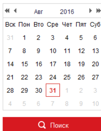
Рисунок 12-2 Поиск видео
