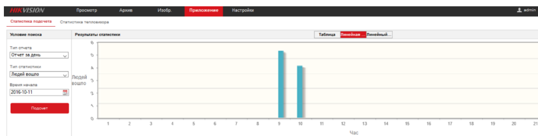
Рисунок 14-2 Подсчет людей
