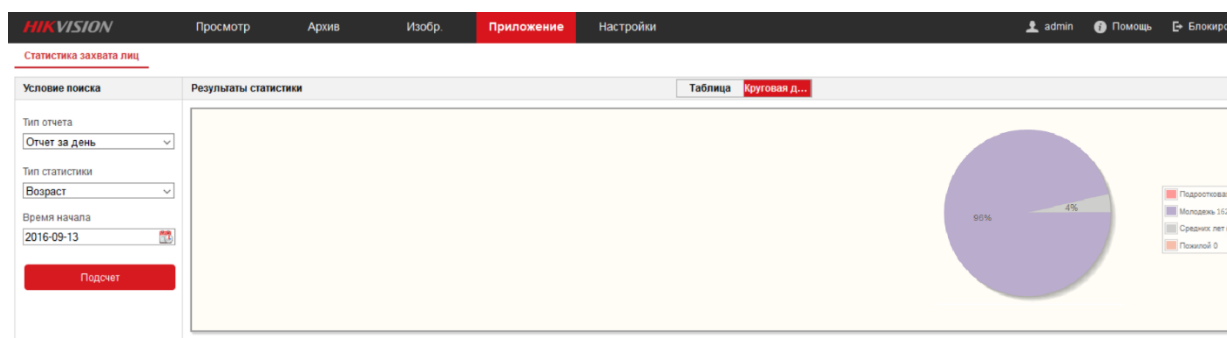
Рисунок 14-1 Интерфейс Приложение
